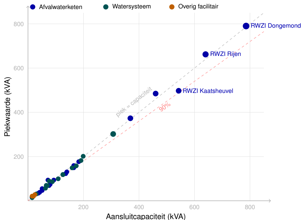
Figuur 1.6: Aansluitcapaciteit versus piekwaarde voor de 38 aansluitingen met meer dan 90% benutting (2025). Punten boven de stippellijn (piek = capaciteit) overschrijden de contractwaarde. De grote RWZI's (afvalwaterketen, rechtsboven) bepalen de absolute vermogensvraag; de overschrijdingen zijn verspreid over alle hoofdgroepen. Bron: Piekanalyse 2025 WSBD.
