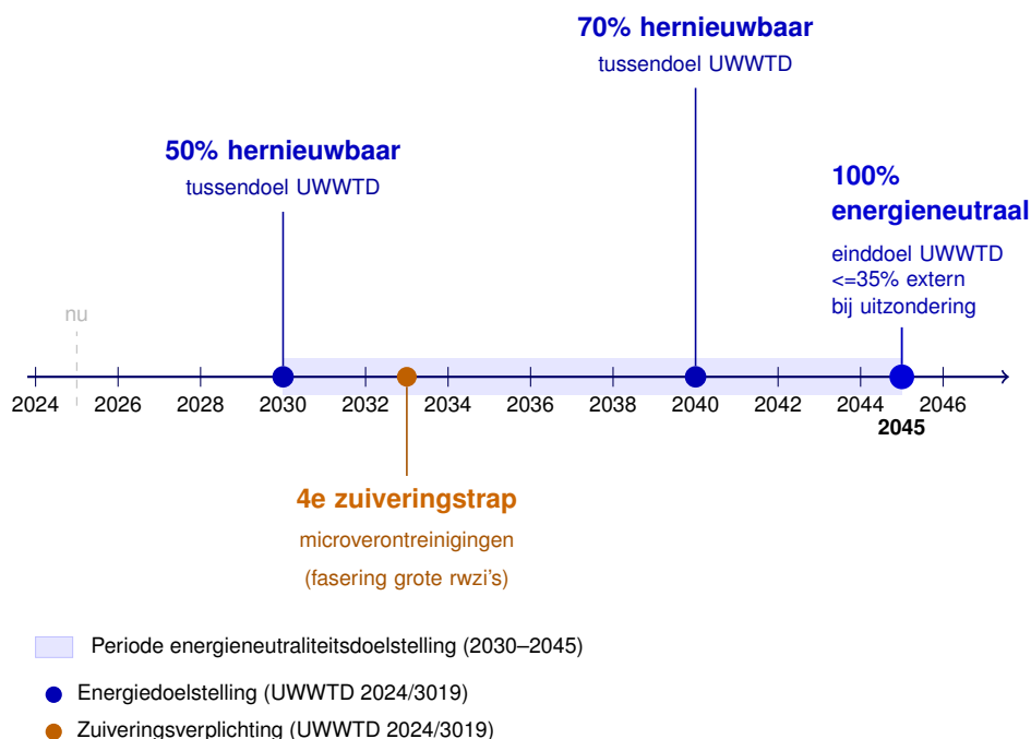
Figuur C.1: Tijdlijn UWWTD-verplichtingen voor de afvalwatersector (Richtlijn 2024/3019/EU). Tussendoelen energieneutraliteit: 50% hernieuwbaar in 2030, 70% in 2040, 100% in 2045. Bij uitzondering mag in 2045 tot maximaal 35% externe niet-fossiele energie worden ingekocht. De vierde zuiveringstrap voor microverontreinigingen verhoogt het energieverbruik van grote rioolwaterzuiveringsinstallaties structureel.
