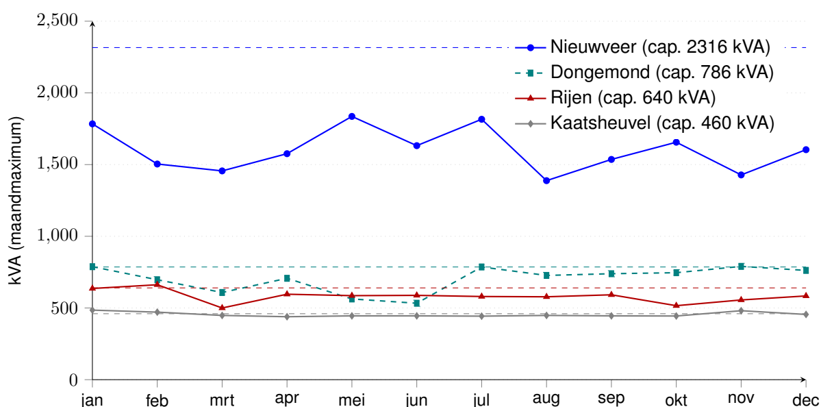
Figuur B.2: Maandelijks piekverbruik (kVA) van de vier grootste RWZI-locaties afgezet tegen aansluitcapaciteit (stippellijn). Bron: Piekanalyse 2025 WSBD.
