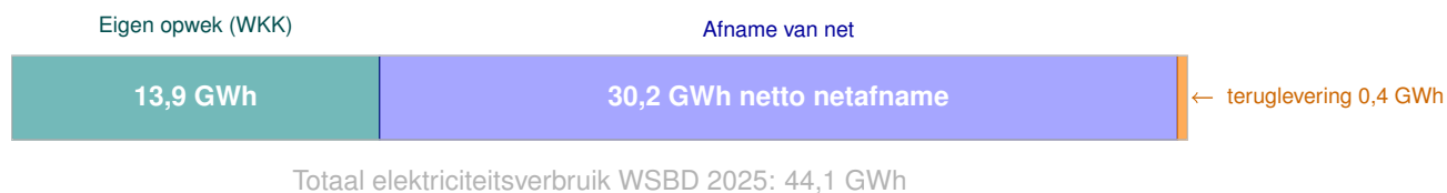
Figuur 1.4: Energiebalans Waterschap Brabantse Delta 2025. De balk toont de samenstelling van het totale elektriciteitsverbruik (44,1 GWh): eigen opwek via warmtekrachtkoppeling (WKK, 13,9 GWh op RWZI Bath, Nieuwveer en Dongemond) en netto afname van het net (30,2 GWh). De teruglevering aan het net bedroeg 0,4 GWh. Bron: meterregistratie WSBD 2025; WKK-productie volgens opgave WSBD (technische reactie, augustus 2026). 4
