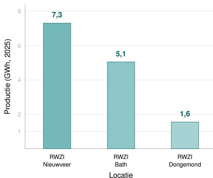
Figuur 1.5: Elektriciteitsproductie via warmtekrachtkoppeling (WKK) per locatie, 2025: RWZI Nieuwveer 7,3 GWh, RWZI Bath 5,1 GWh en RWZI Dongemond 1,6 GWh (totaal 13,9 GWh). De WKK-productie draait achter de meter en is daarom niet volledig zichtbaar in de meterregistratie. Bron: opgave WSBD (technische reactie, augustus 2026).
