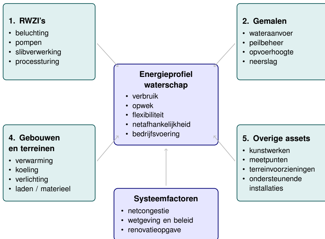
Figuur A.1: Relatie tussen assetcategorieën, energieverbruik, opwekking en netafhankelijkheid. Kwalitatief overzicht; geen kwantitatieve verdeling naar energieverbruik. De indeling volgt de vijf hoofdgroepen die in dit onderzoek worden gehanteerd (paragraaf 1.2.2) en sluit aan op de indeling naar hoofdgroep assets in de meterregistratie van het waterschap.
