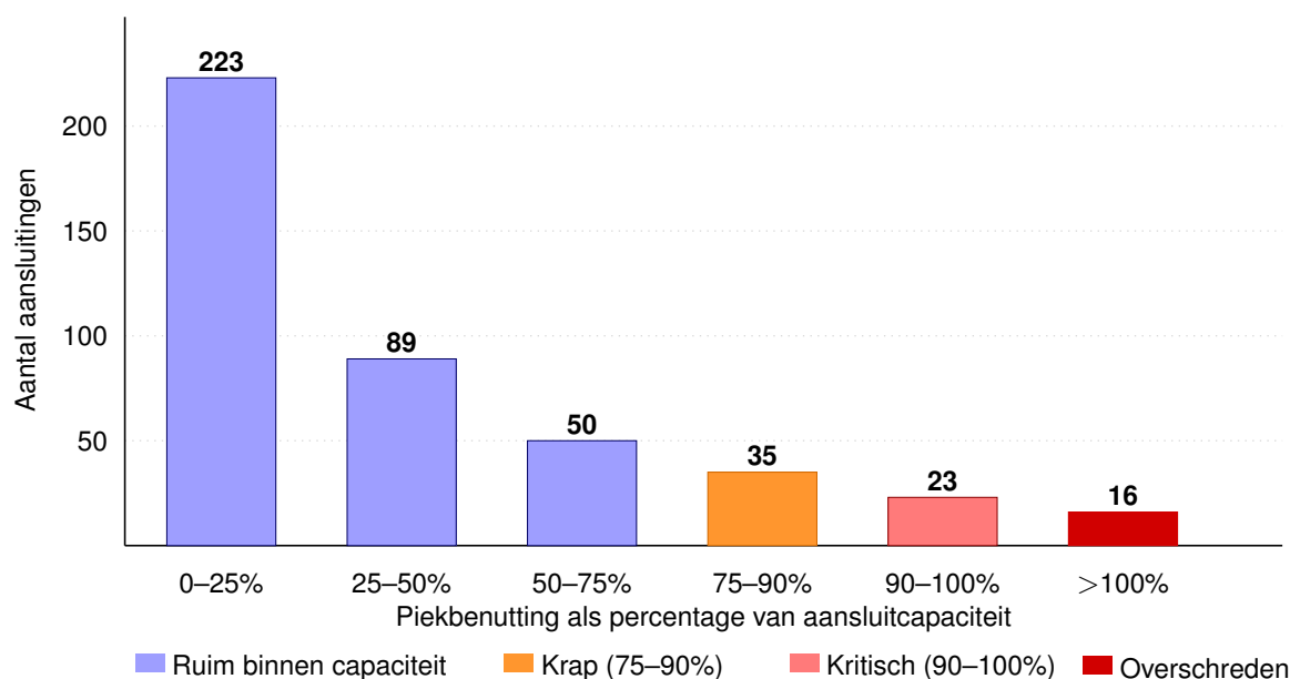
Figuur B.1: Verdeling piekbenutting van de aansluitcapaciteit over 436 actieve elektriciteitsaansluitingen (2025). Kleur geeft urgentieniveau aan. Bron: Piekanalyse 2025 WSBD (Piekanalyse_2025_WSBD.xlsx).
